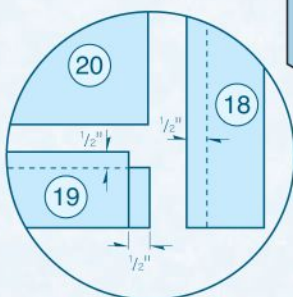
Door Tenon and Groove Detail
